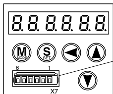
连接器 X7 制造厂型号：530140610 制造厂：Molex株式会社
