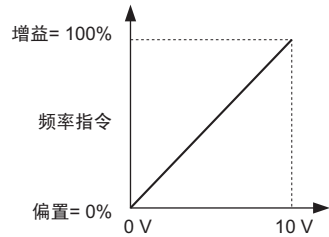
图 5.25 模拟量输入端子 A1 的特点（出厂设定）
