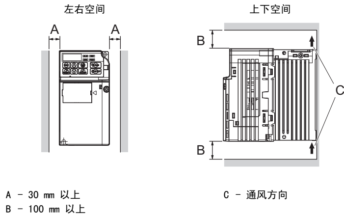
图 2.2 变频器的安装空间（单机） （注）柜内安装型（IP20）和封闭壁挂型（NEMA Type1）所需的上下、左右空间均相同。
