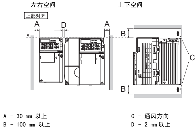
图 2.3 变频器的安装空间（并列） （注）并列安装大小不同的变频器时，请对齐各变频器的上部位置再进行安装。否则，更换冷却风扇时将无法拆下风扇。
