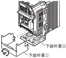
图 8.12 下部外罩的拆卸方法
